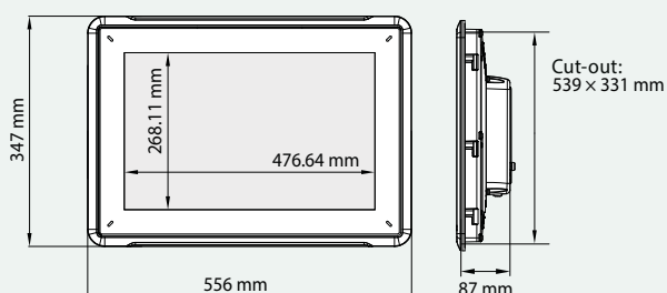
15" Web Panel PCD7.D5150WTA010 PCD7.D6150WTA010
